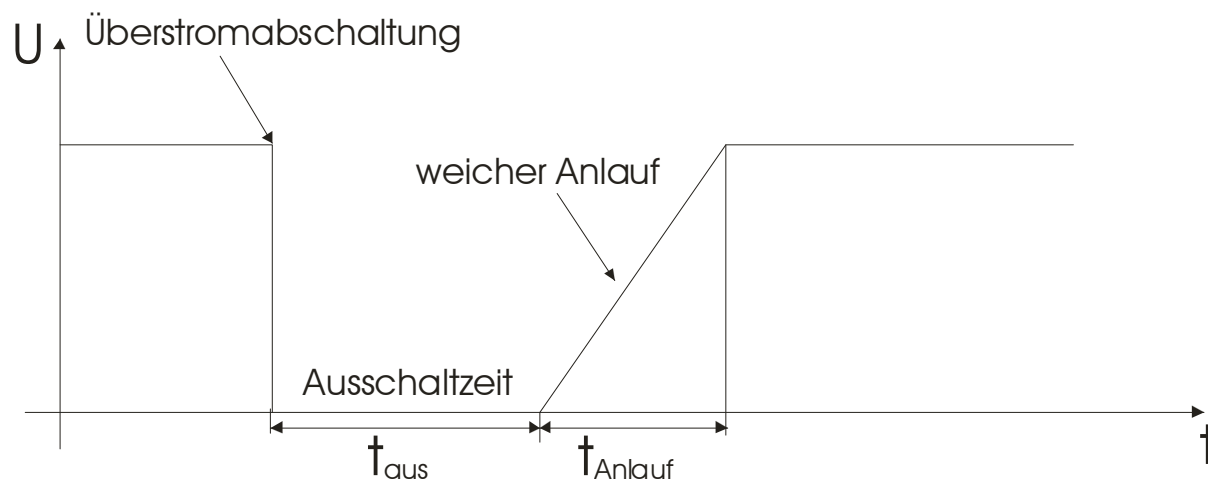
Abbildung 1: Überstromabschaltung
