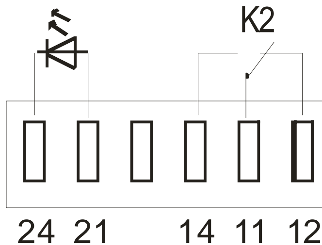
Abbildung 4: Klemmenbelegung
